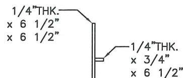
S.S. TEE BKT DTL.
